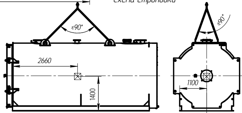
Схема строповки
