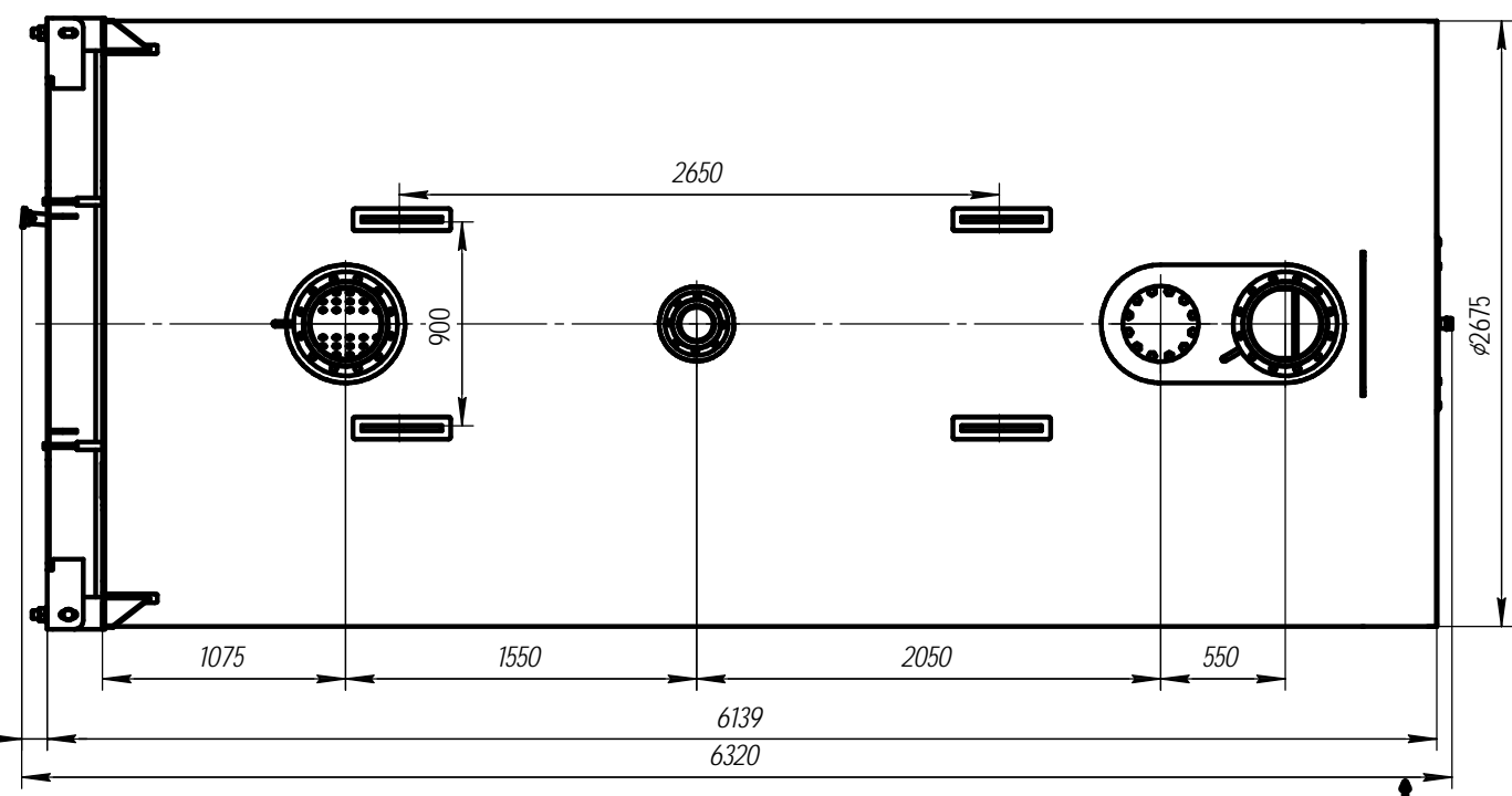
Схема строповки
